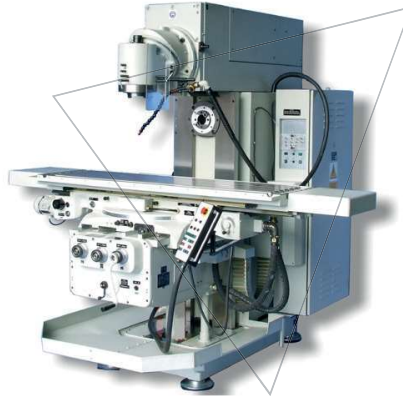
Universalfräsmaschine FU450MRAPuG
