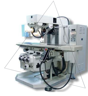
Horizontalfräsmaschine FW450MR
